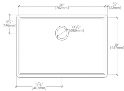
TOP VIEW SCALE: 1"=1'-0"
