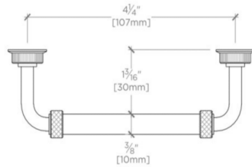
TOP VIEW SCALE: 6"=1'-0"
