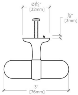
TOP VIEW SCALE: 6"=1'-0"
