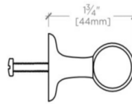
SIDE VIEW SCALE: 6"=1'-0"
