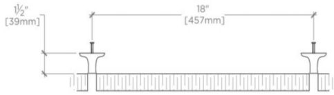
TOP VIEW SCALE: 1 1/2"=1'-0"
