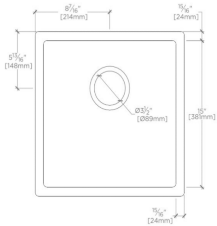
TOP VIEW SCALE: 1\frac{1}{2}"=1'-0"
